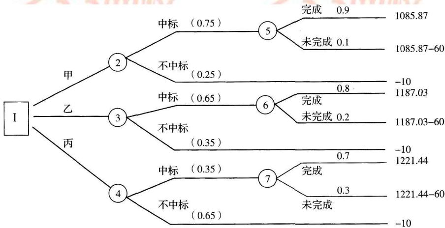
图 4-3 决策树
