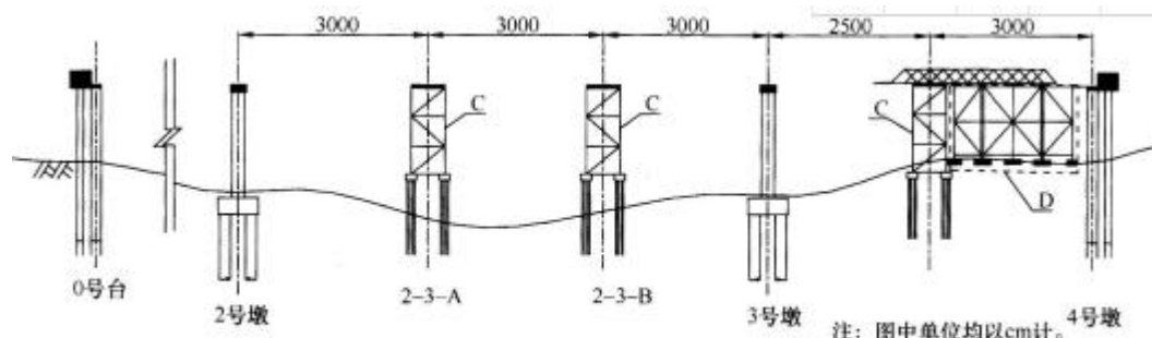
图 5 主桥桥跨与主梁钢桁梁拼装顶推现场布置图
