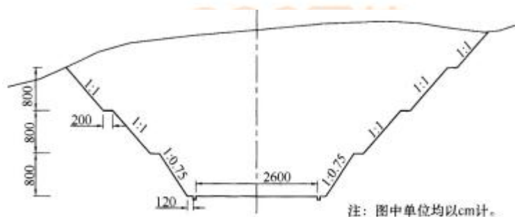
图 3 K18+520 横断面设计示意图
