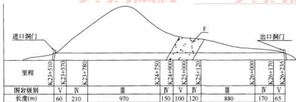
图 1 隧道纵断面示意图
