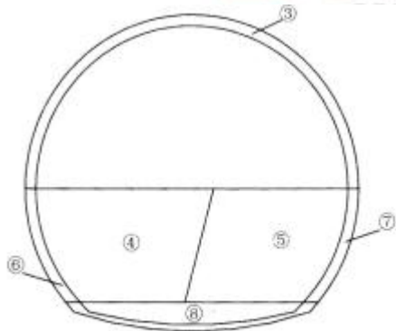
图 2 隧道开挖横断面示意图
