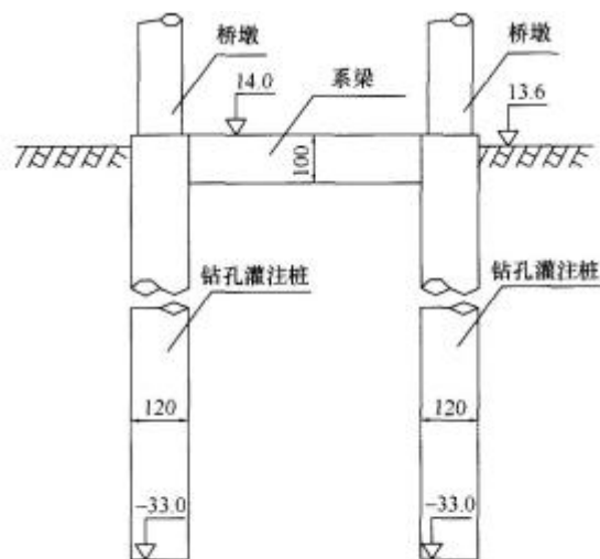
图 7 某桥墩桩基立面示意图
