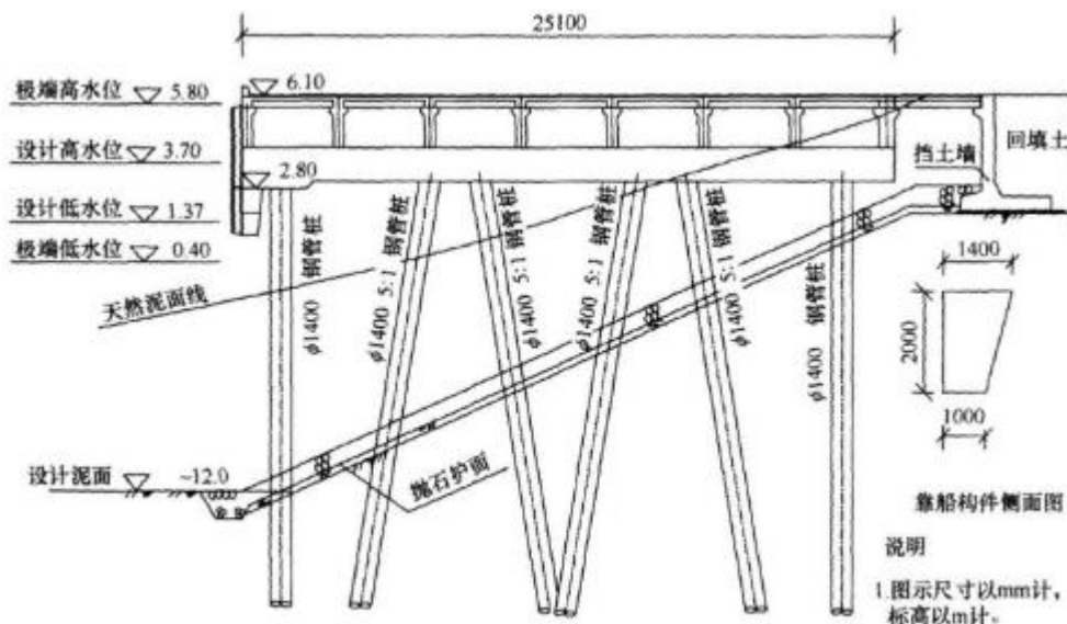
图 1 码头断面图
