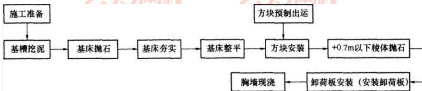
图 6 开工到胸墙浇筑的施工流程框图
