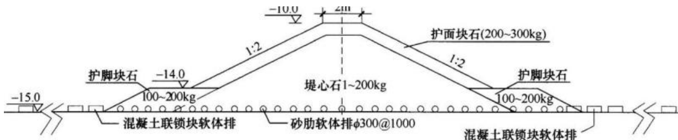
图 2 典型断面示意图
