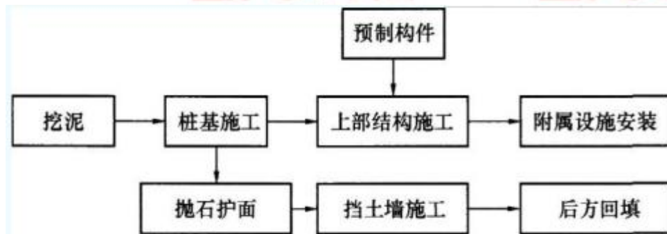
图 4 施工流程框图
