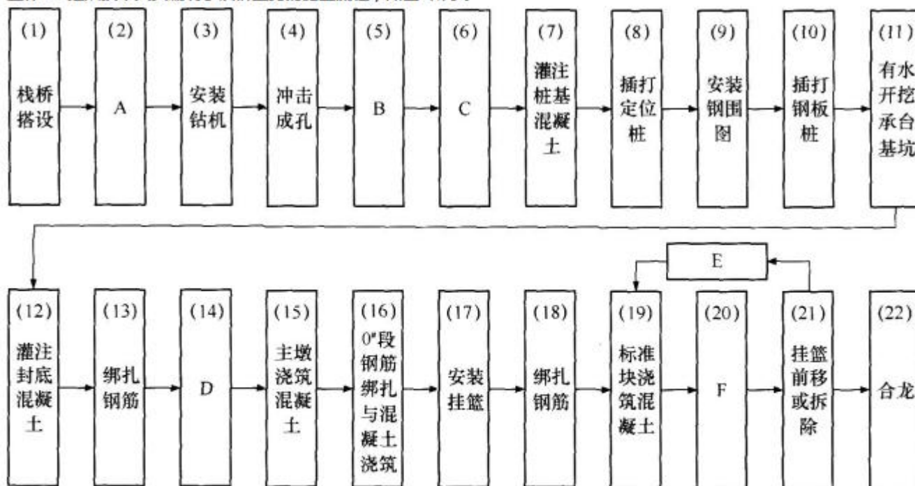
图 3 主跨桥施工流程图
