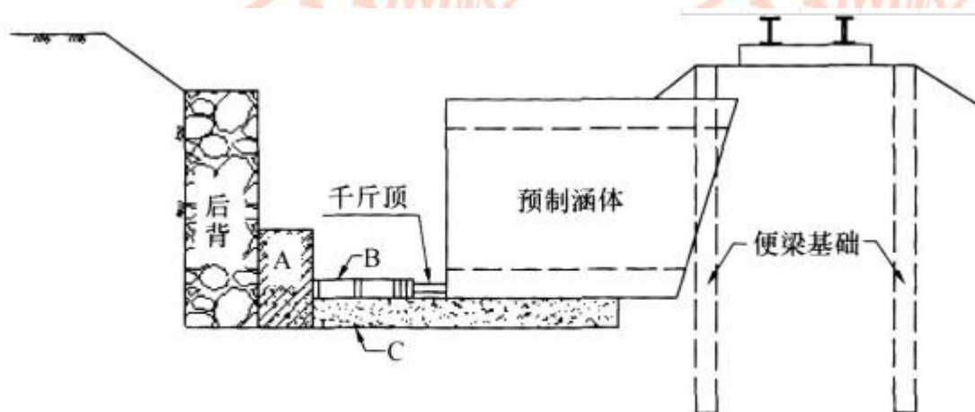
图 6 交通涵顶进施工示意图
