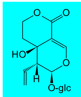
獐牙菜苦苷
