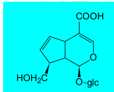
京尼平苷酸
