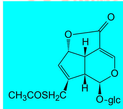
鸡屎藤苷
