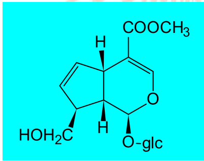
栀子苷
