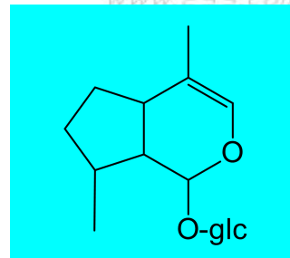
环烯醚萜苷
