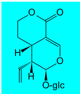
獐牙菜苷
