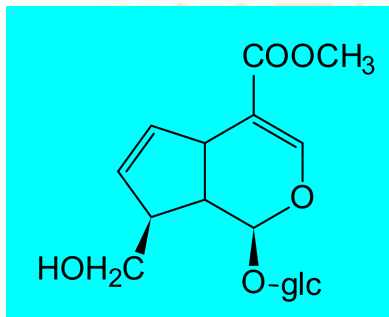
京尼平苷
