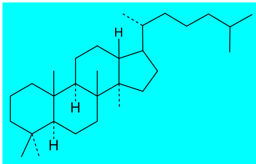
达玛烷
