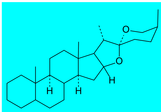
螺旋甾烷
