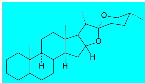
异螺旋甾烷
