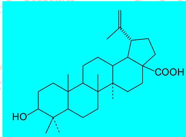
异螺旋甾烷
