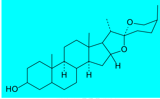
菝葜皂苷元
