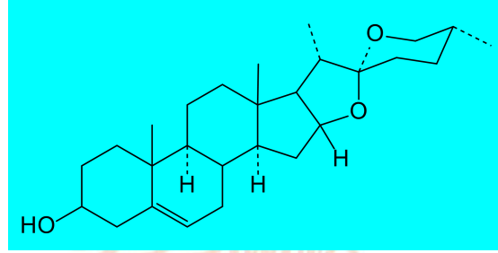
薯蓣皂苷元
