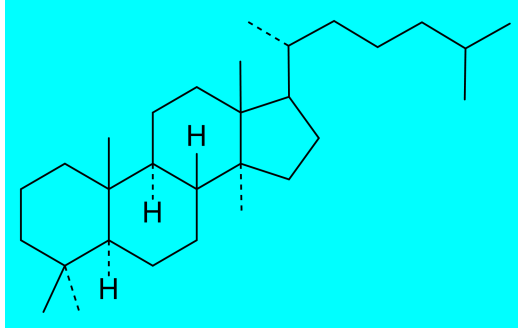
羊毛甾烷
