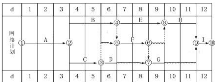
室内装饰工程时标网络计划图 (时间单位: 周)
