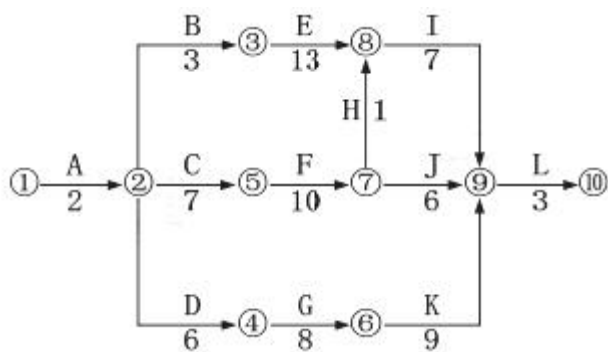
图 1 施工进度计划网络图（时间单位：周）
