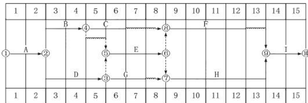
室内装饰工程时标网络计划图 (时间单位: 周)
