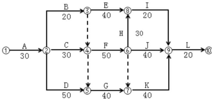
图4-1 施工网络进度计划（单位：天）
