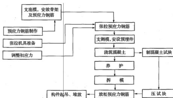
图 4.1.27 先张法工艺流程
